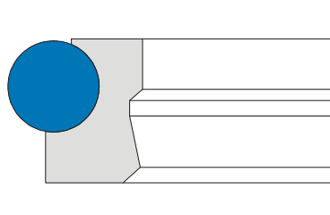
Pierścień zgarniający ZD-05
