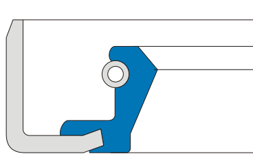
Uszczelnienie wału UW-B
