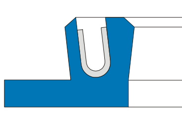
Pierścień rowkowy wału UW-PR
